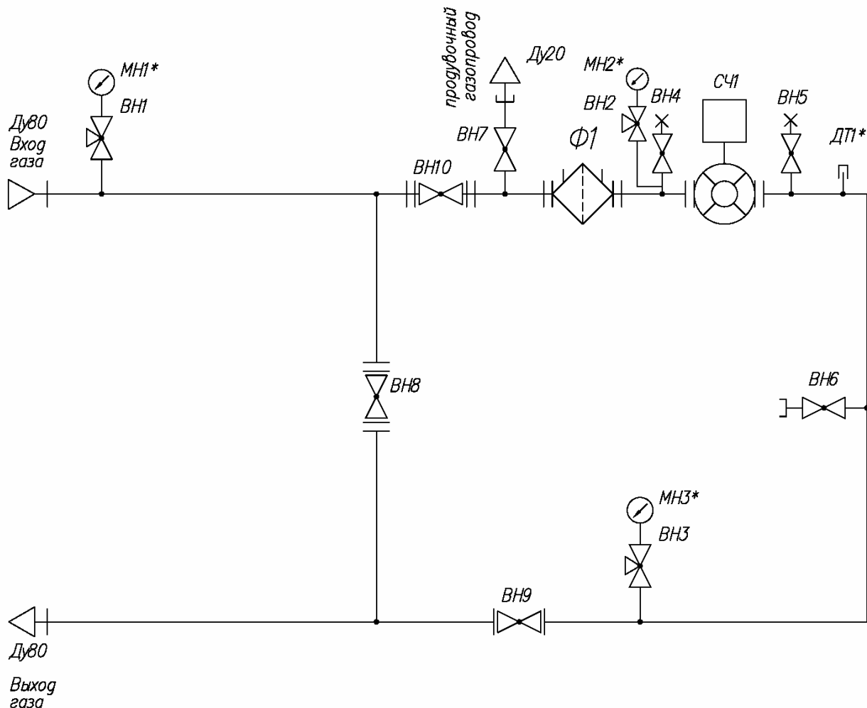
Схема принципиальная.
